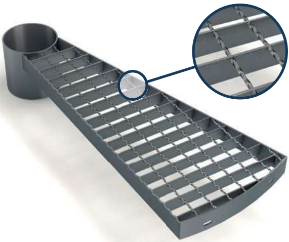
Schweisspressroste Maschenweite: 34 x 38 mm
